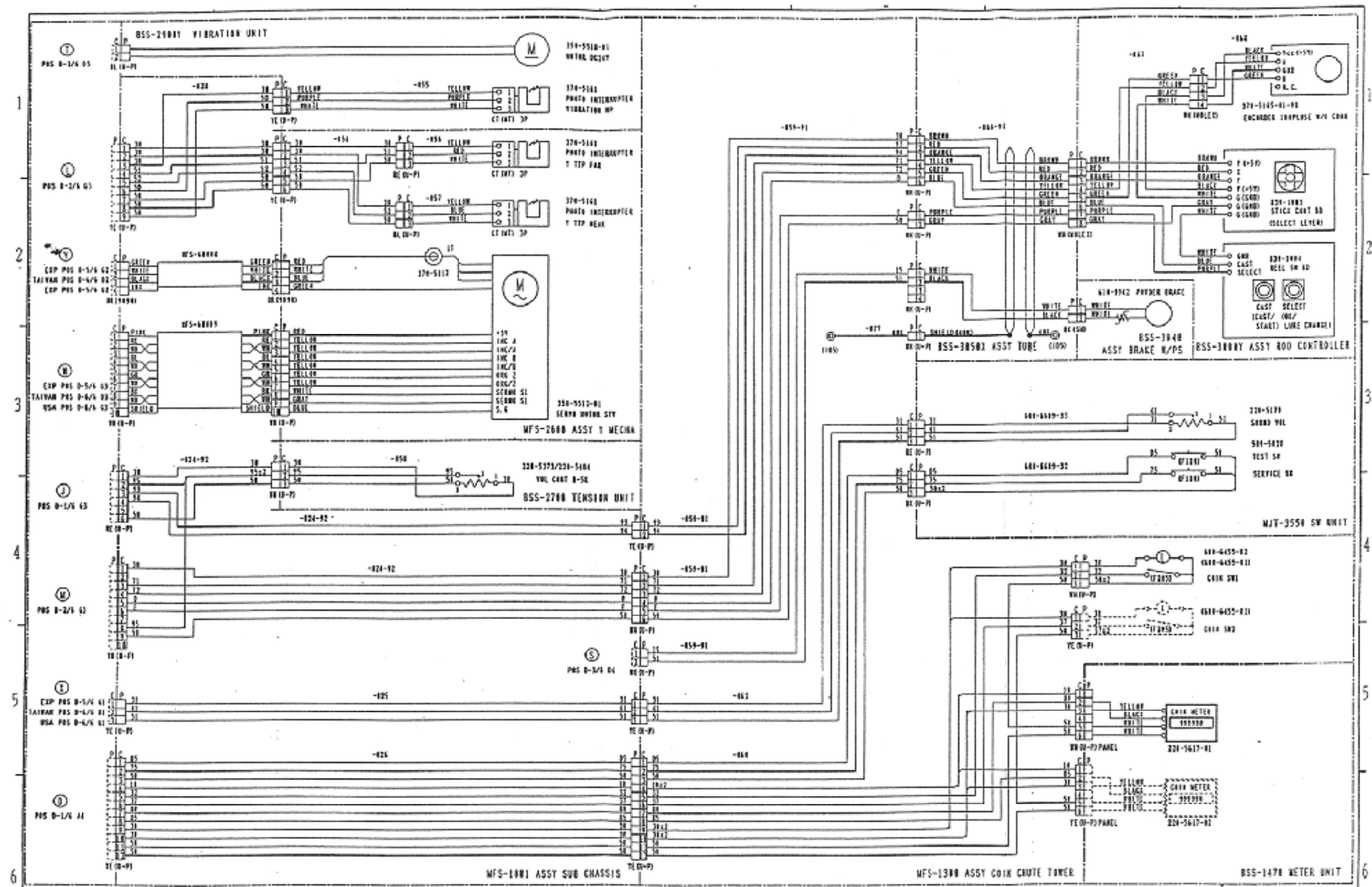
20. WIRING DIAGRAM (D-4/6)
