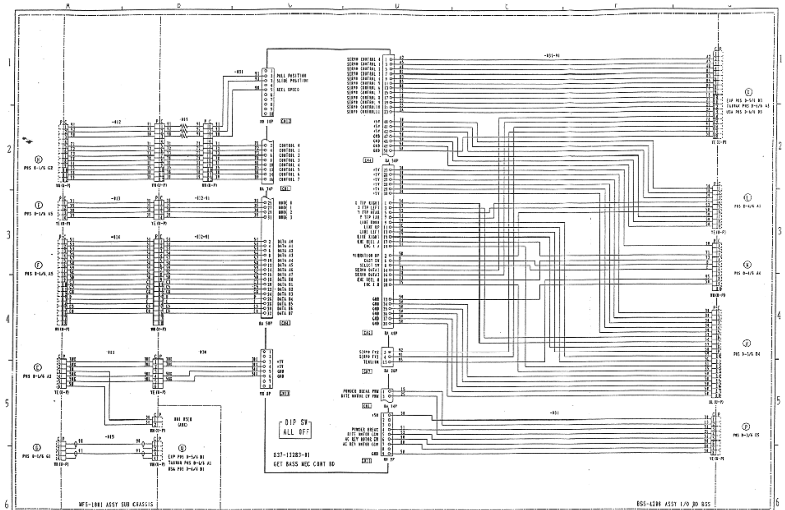
20. WIRING DIAGRAM (D-2/6)
