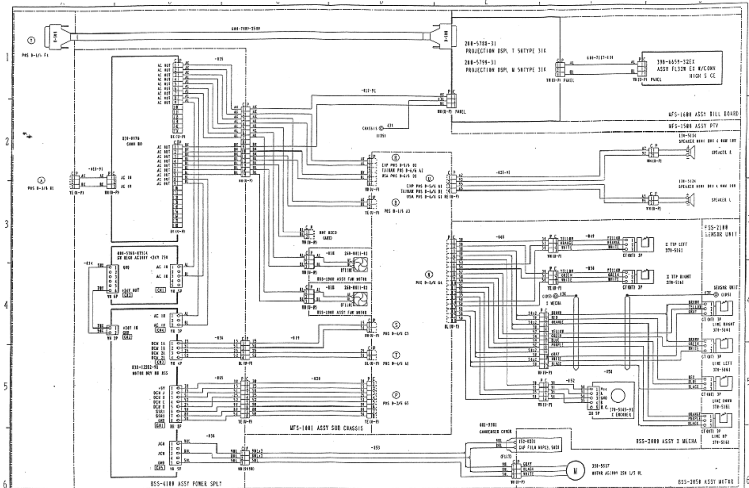
20. WIRING DIAGRAM (D-3/6)
